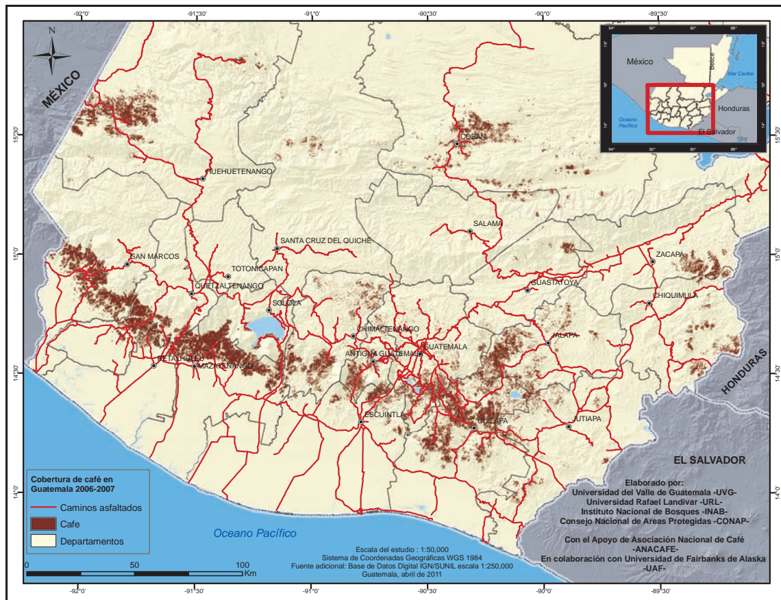
Figura 11. Mapa de la cobertura de café para Guatemala al año 2006.
