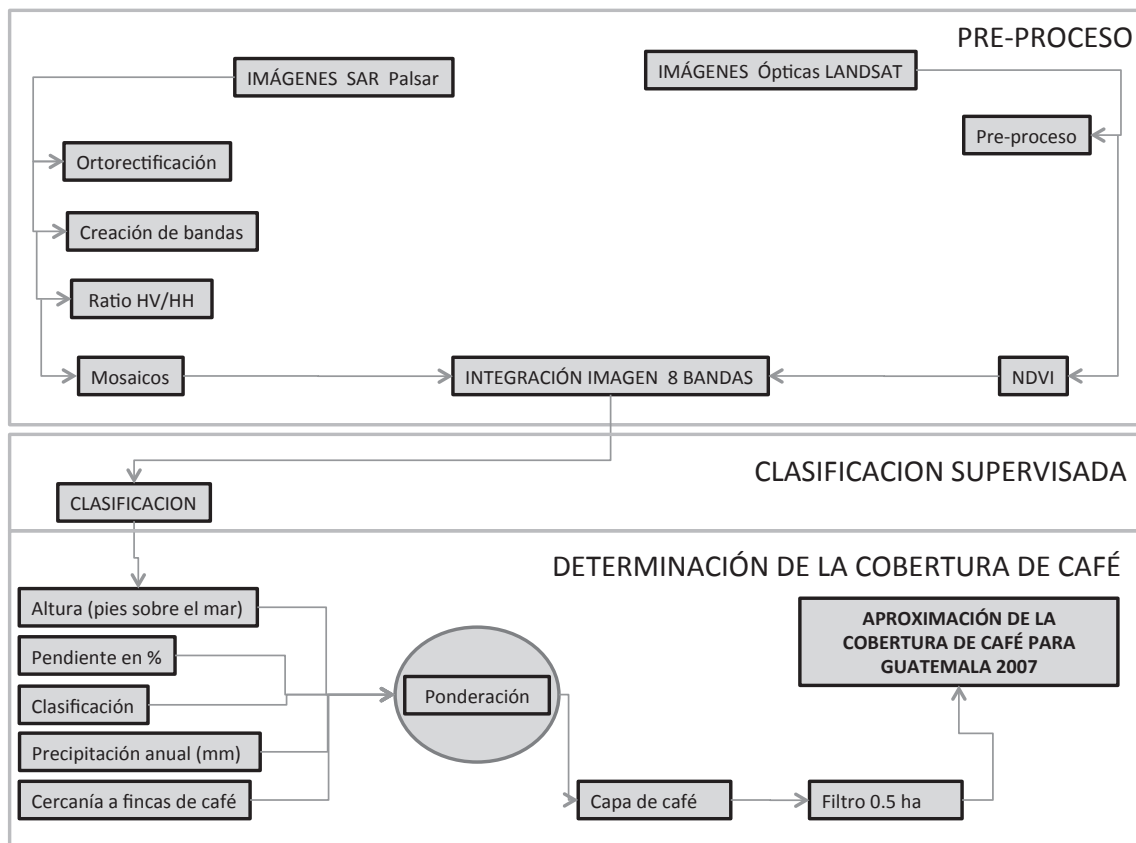
Figura 10. Diagrama de flujo de la secuencia de procedimientos desarrollados para obtener una aproximación de la cobertura de café para la República de Guatemala.
