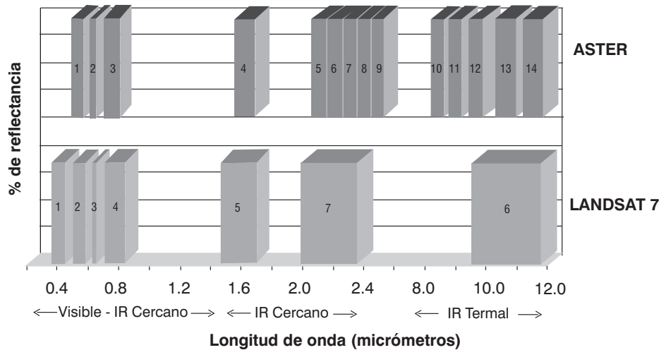
Figura 1. Comparación entre datos colectados por sensores ASTER y LANDSAT 7.
